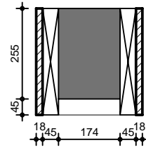
VUE EN COUPE AA
