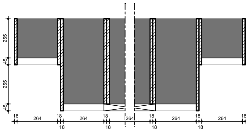
VUE EN COUPE DD
