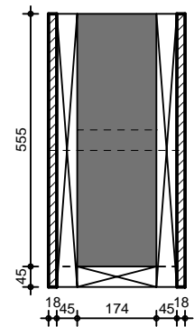
VUE EN COUPE CC
