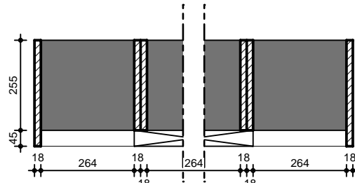
VUE EN COUPE CC
