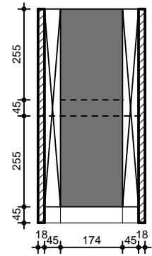
VUE EN COUPE BB
